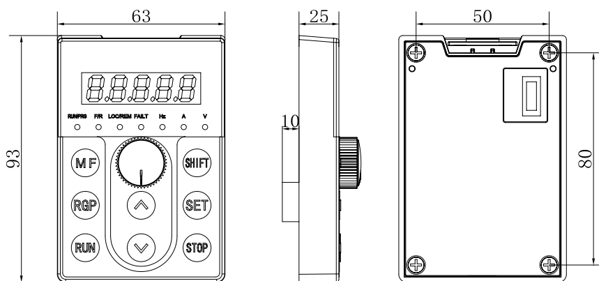
Рисунок 5.6. Панель управления
