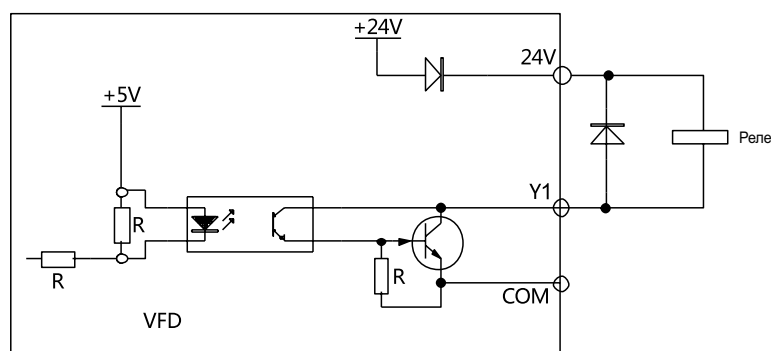
Рисунок 4.17. Схема подключения клеммы многофункционального выхода, режим 1
