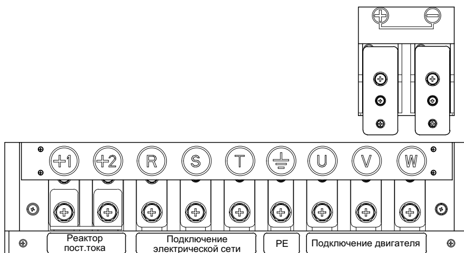
Рисунок 4.10. Силовые клеммы NVF2G-160/TS4-315/PS4
