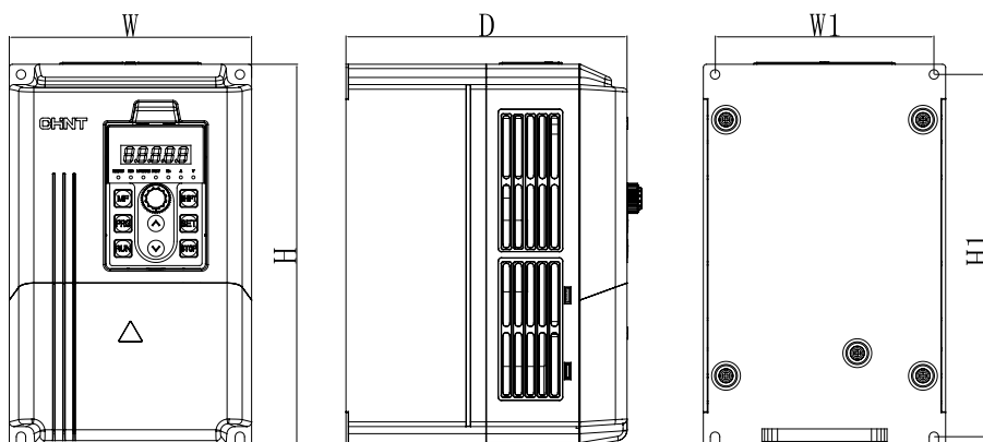
Рисунок 5.1. Внешний вид и габаритные размеры NVF2G-1.5/PS4–NVF2G-11/PS4
