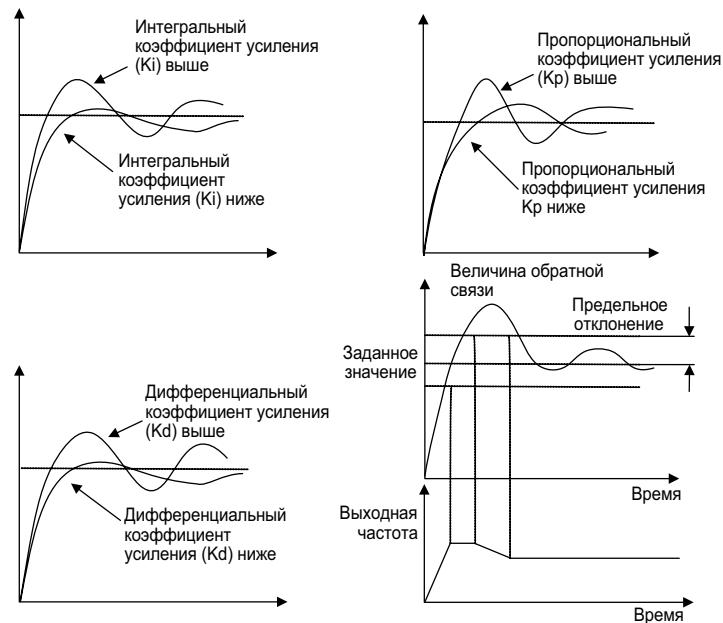
Рисунок 8.2.8. Влияние параметров ПИД-регулятора
