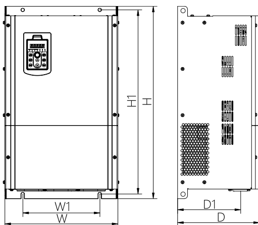
Рисунок 5.3. Внешний вид и габаритные размеры NVF2G-30/PS4–NVF2G-75/PS4
