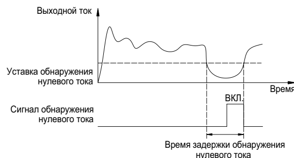
Рисунок 8.18.1. Принципиальная схема обнаружения нулевого тока
