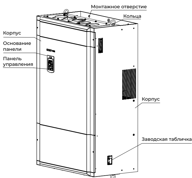
Рисунок 4.5. Внешние компоненты NVF2G-315/TS4–NVF2G-400/TS4
