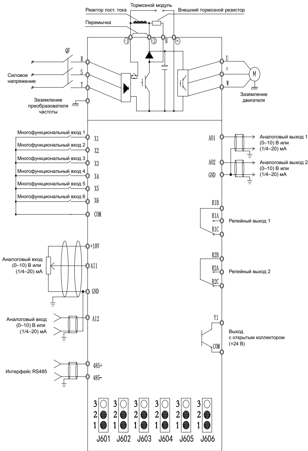
Рисунок 4.12 Схема подключения NVF2G-1.5/PS4–NVF2G-400/TS4
