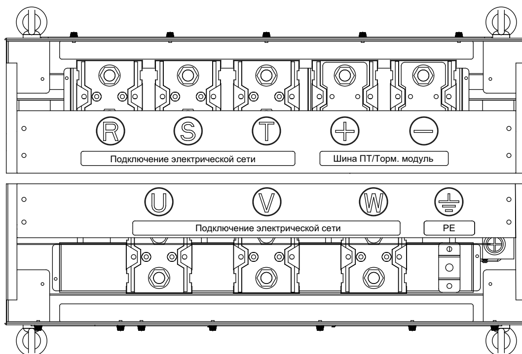
Рисунок 4.11. Силовые клеммы NVF2G-315/TS4-400/TS4
