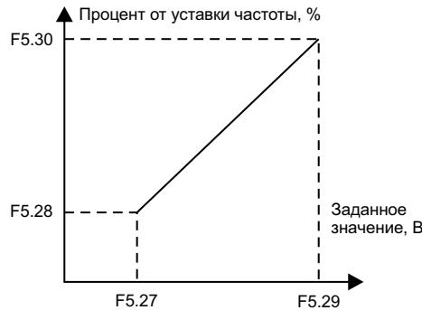
Рисунок 8.2.1. Настройка кривой аналогового входа 1
