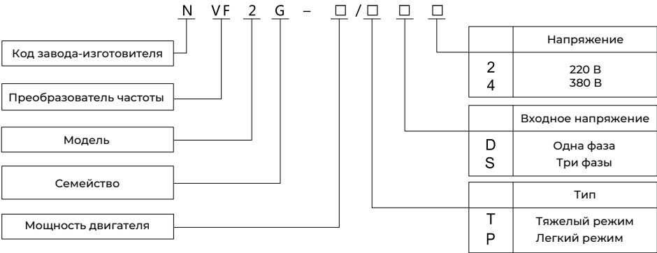
Рисунок 1.2. Расшифровка заводской таблички
