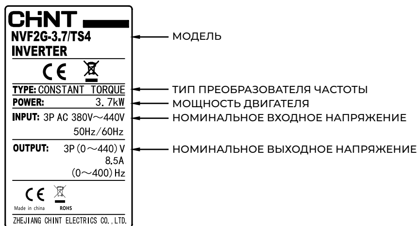
Рисунок 1.1. Заводская табличка устройства
